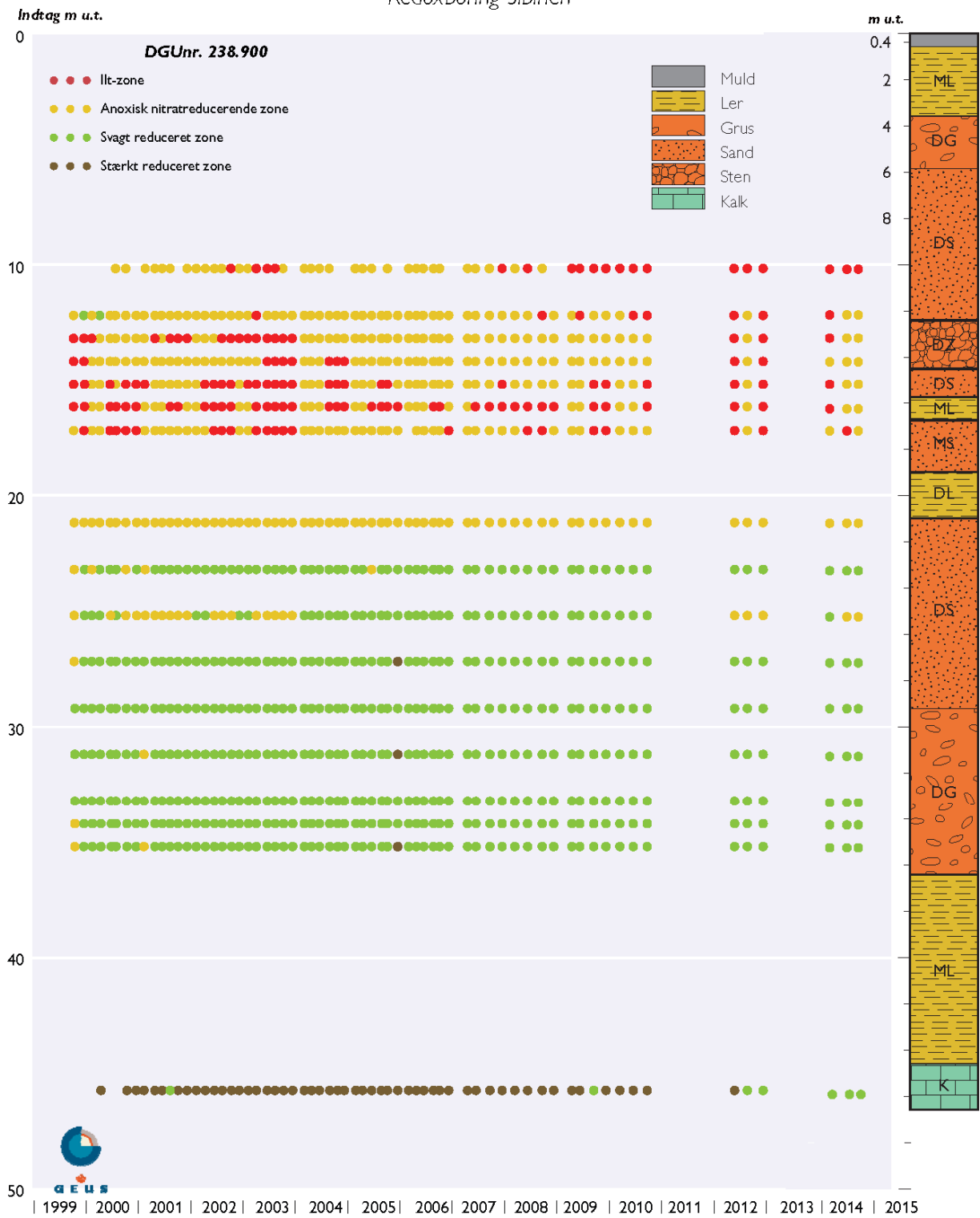
Figur 18. Redoxzoner 10 - 46 m u.t. for redoxboring DGU nr. 238.900, Sibirien på Falster, 2000-2014. Grundvandsspejl i ca. 8-9 m u.t. Den geologiske lagserie er vist længst til højre.
