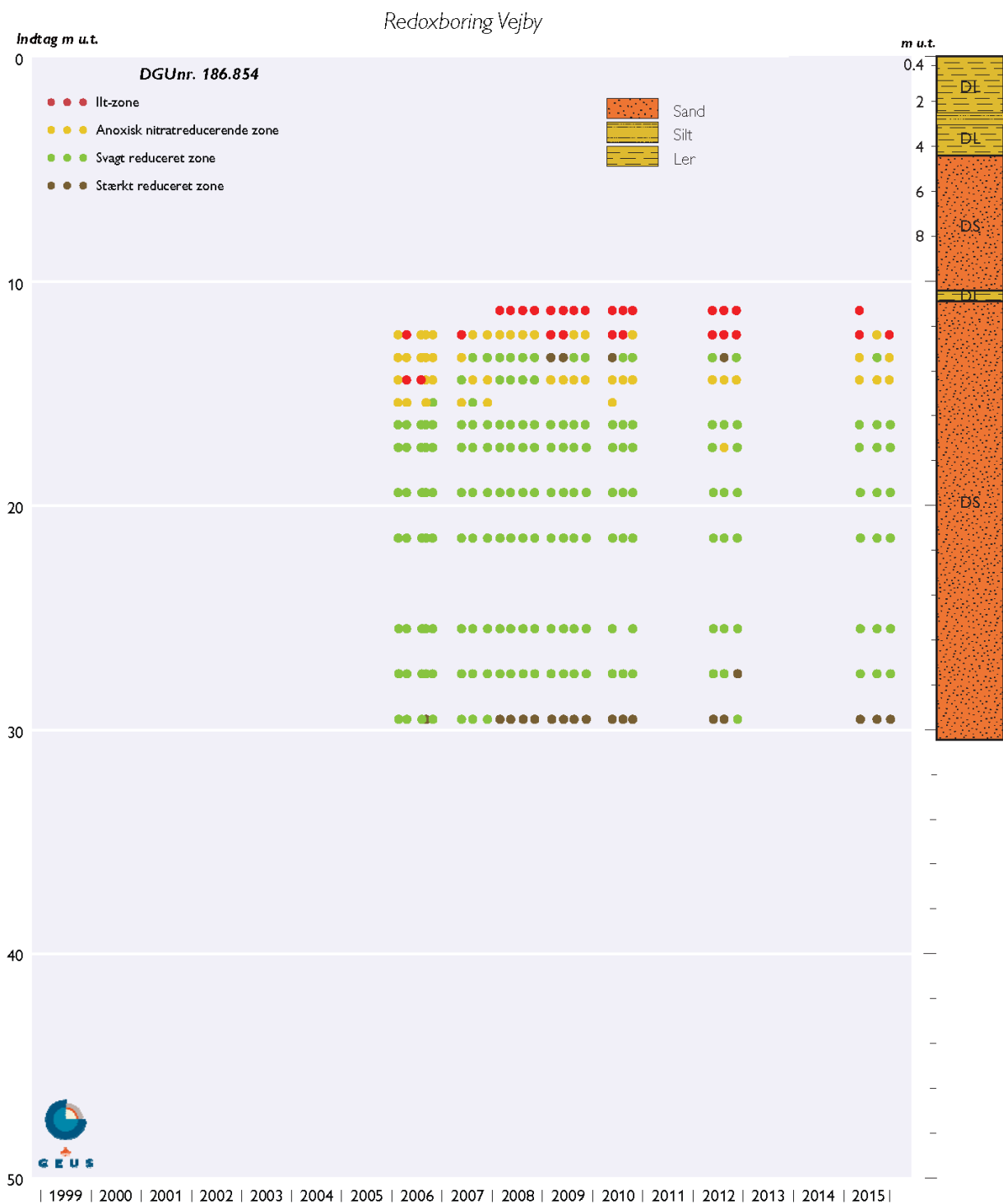
Figur 19. Redoxzoner 13 - 30 mu.t. for redoxboring DGU nr. 186.854 og 186.855, Vejby, Nord-sjælland, 2006-2014. Grundvandsspejl i ca. 10 m u.t. Den geologiske lagserie er vist til højre.
