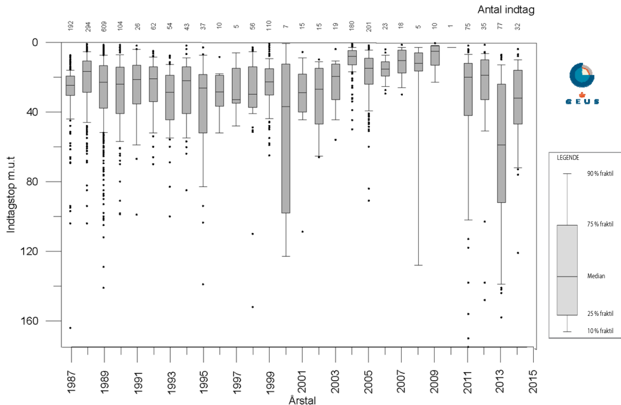
Figur 5. Dybdefordeling af afstanden fra terræn til overkanten af indtaget for nye indtag i overvågningen som funktion af det år, de i JUPITER angives til at indgå i GRUMO-stationsnettet. Medianværdien er vist med en vandret streg. Boksen repræsenterer de midterste 25-75 % af fordelingen de enkelte år. 80 % af indtagene ligger inden for linjen. Øverst er angivet antal nye indtag for hvert enkelt år.
